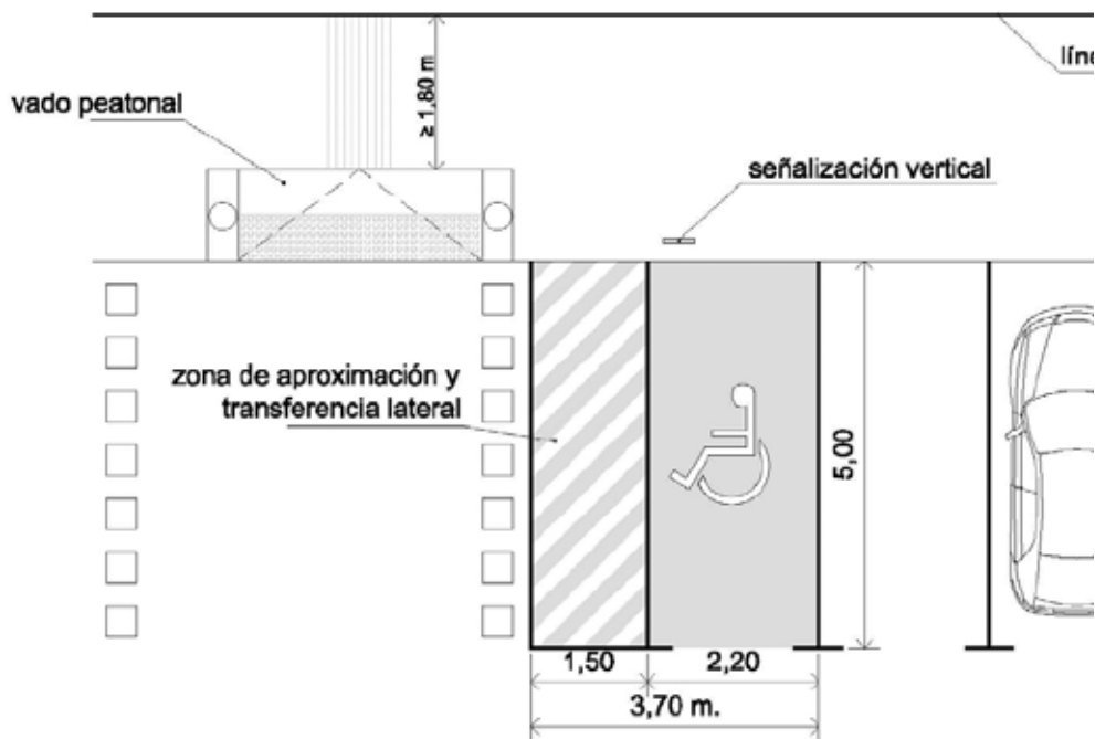
Figura 2. Plaza de aparcamiento reservada con acceso desde paso de pe
